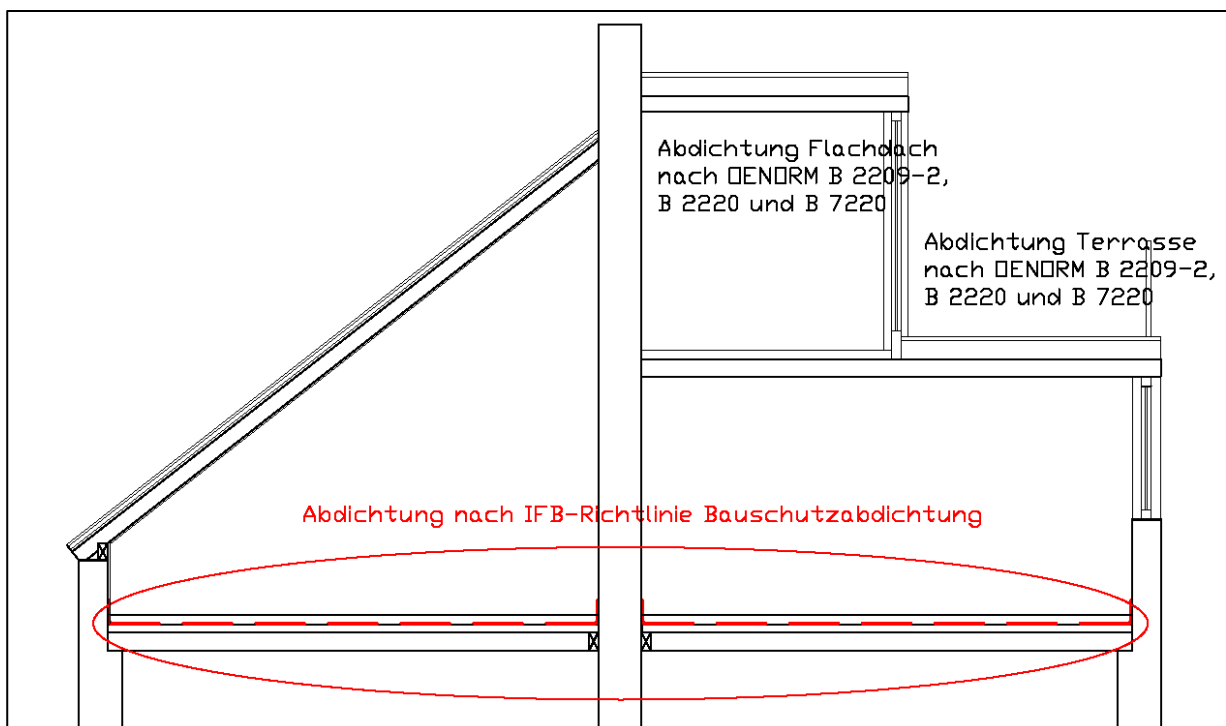
Abb.1: Anwendungsbereich Richtlinie Bauschutzabdichtung
