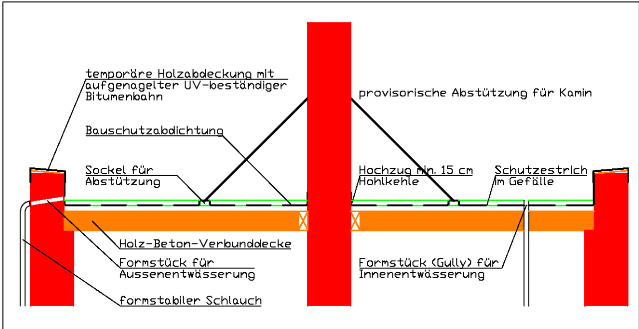
Abb. 7: Systemskizze
